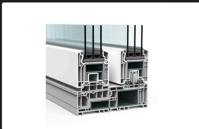
Umlaufende Stahlverstärkungen in Rahmen und Flügeln
